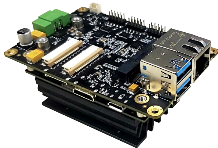
与 Xavier_nx 模组实物连接图
